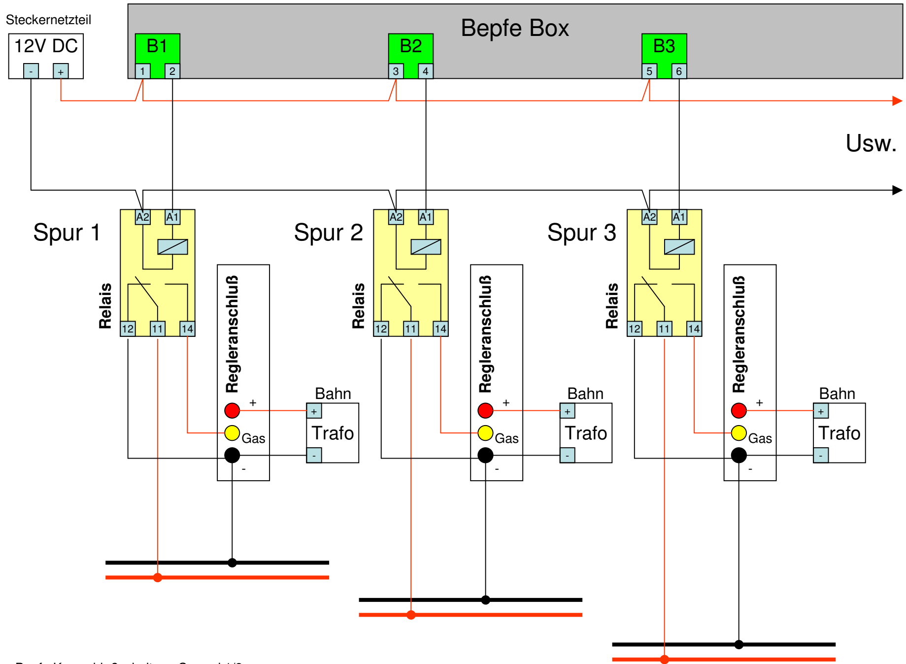
Bepfe Kurzschlußschaltung Conrad 1/2
